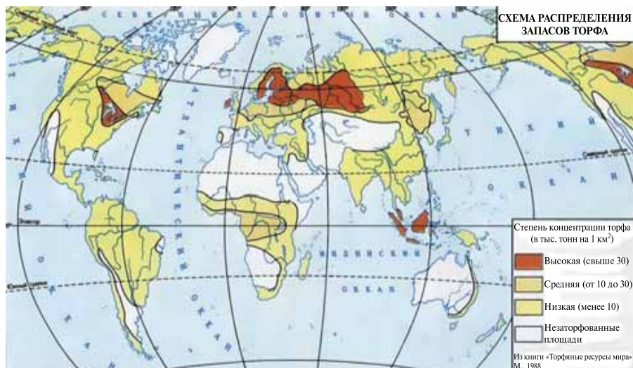
Рис. 23. Схема расположения торфяников на планете
