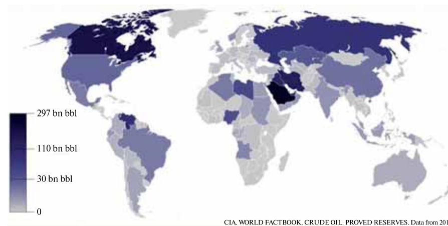
Рис. 25. Схема месторождений нефти на планете
