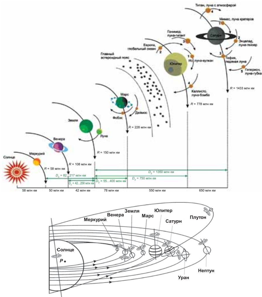
Рис. 4. Совмещенная схема движения планет Солнечной системы, спутников планет и вращения планет вокруг собственных осей
