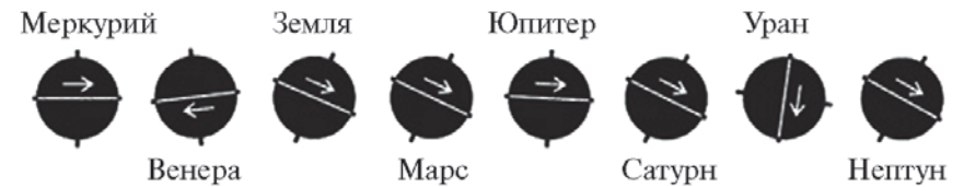
Рис. 293. Направления вращения планет Солнечной системы вокруг своей оси
