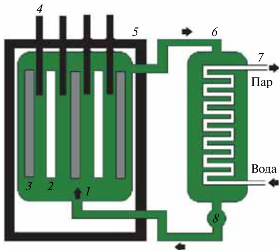
Рис. 181. Схема работы атомного энергоблока:
