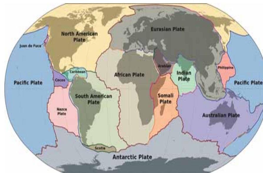
Рис. 240. Основные тектонические плиты литосферы Земли
