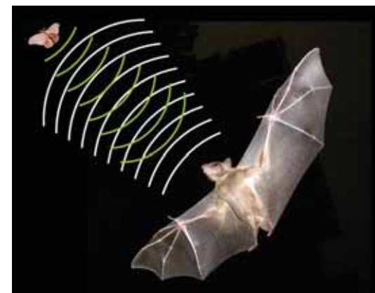
Рис. 54. Использование эхолокации летучей мышью
