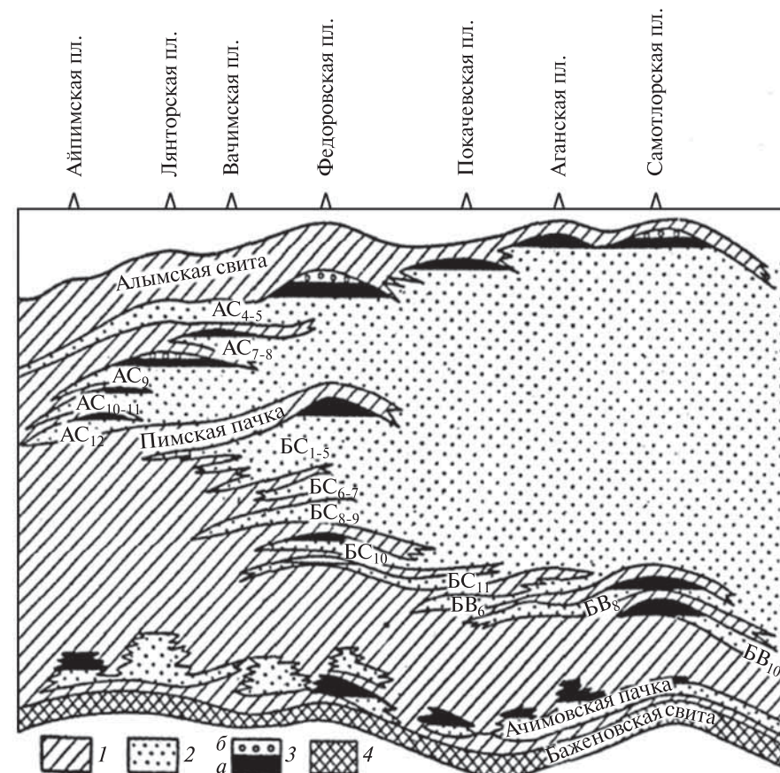
Рис. 38. Схематический геологический профиль отложений Среднего Приобья [5]:
