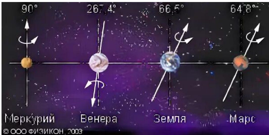
Направление вращения Меркурия и планет земной группы
