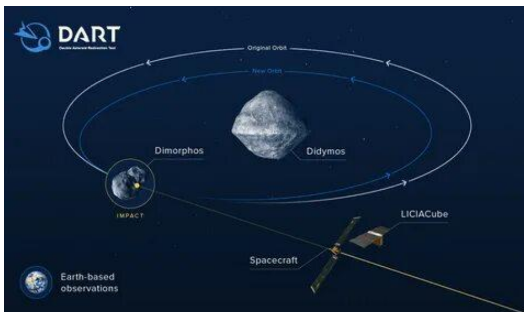
Столкновение космического аппарата с астероидом Диморф
